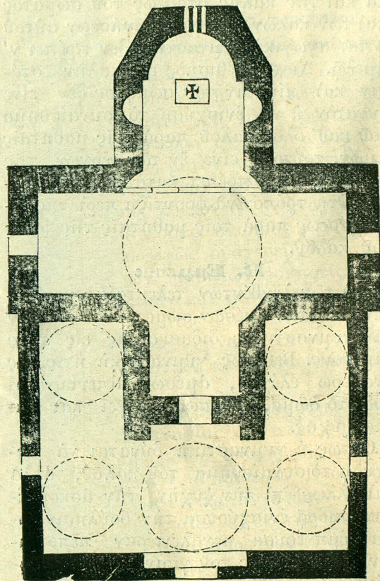
(Εἰκ. 17). Ἀρχιτεκτονικὴ κάτοψις τοῦ ἐν Μανωλάδι παρὰ τὴν Ἀχαΐαν ναοῦ τῆς Θεοτόκου.
