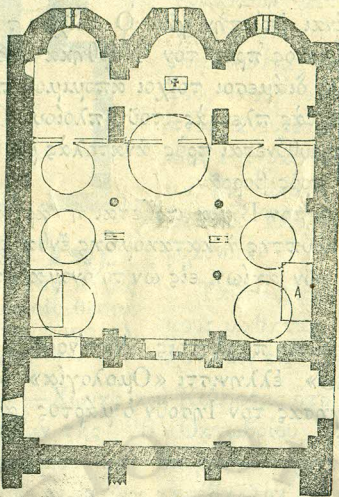
(Εἰκ. 10). Ἀρχιτεκτονικὴ κάτοψις τοῦ παρὰ τὴν Ἄρταν ναοῦ τῆς Μονῆς Βλαχερνῶν.
