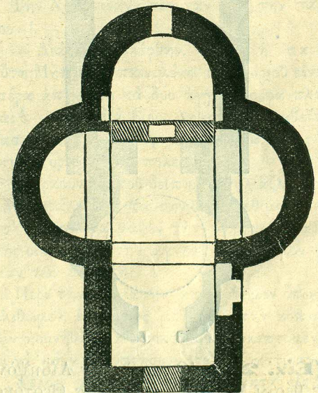
(Εἰκ. 21). Ἀρχιτεκτονικὴ κάτοψις τοῦ ναοῦ τοῦ ἐν Μεθάνοις ναοῦ τοῦ Αγίου Νικολάου.
