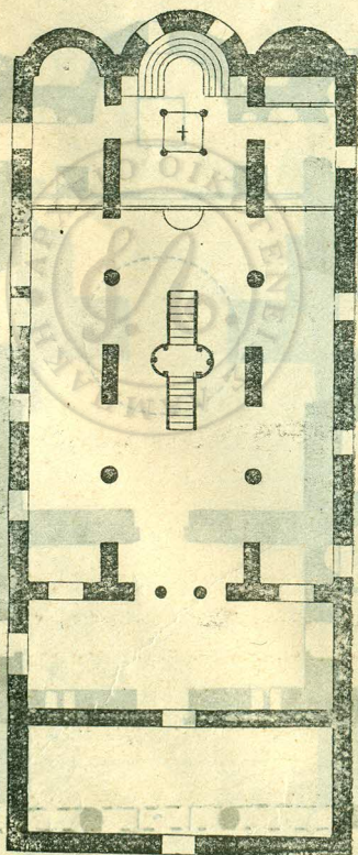
(Εἰκ. 24). Ἀρχιτεκτονικὴ κάτοψις τοῦ Μητροπολιτικοῦ ναοῦ Σταγῶν (Καλαμπάκα) ἐν μέσῳ τοῦ ὁποίου κεῖται ὁ ἄμβων.
