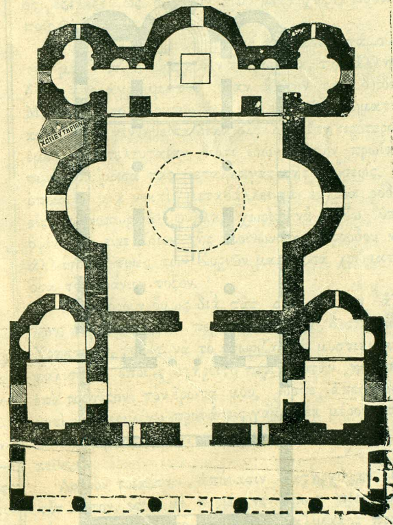
(Εἰκ. 22). Ἀρχιτεκτονικὴ κάτοψις τοῦ παρὰ τὴν Ὑπάτην ναοῦ τῆς Μονῆς Αγάθωνος, ἐκατέρωθι τοῦ ἔσω νάρθηκος ἔχοντος δύο παρεκκλήσια.
