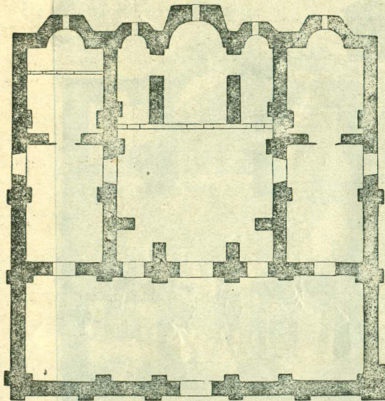
(Εἰκ. 7). Ἀρχιτεκτονικὴ κάτοψις τοῦ ἐν ᾿Αοτῇ ναοῦ τῆς Παρηγορητίσσης.
