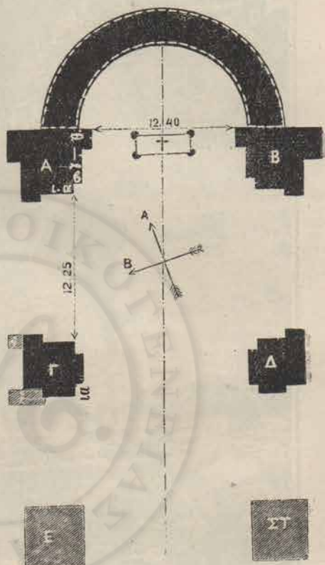
Εἰκ. 180. Ἀρχιτεκτονικὴ κατόψις τοῦ ἐν Φιλαδελφείᾳ ἡρειπωμένου Ναοῦ, Ἰωάννου τοῦ Θεολόγου.
