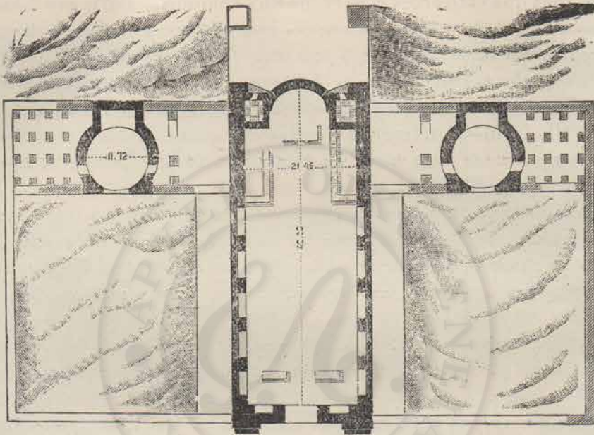
Εἰκ. 143. Ἀρχιτεκτονικὴ κάτοψις τῆς ἐν Περγάμῳ Βασιλικῆς, μετὰ τῆς ἐαυτῆς περιοχῆς. (Texier. II. pl. 118.).
