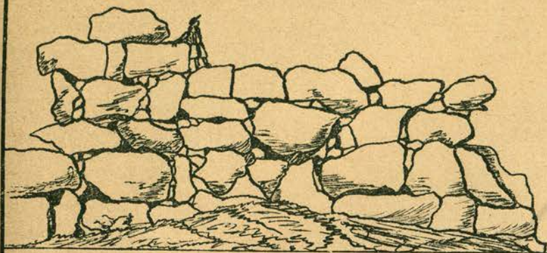
1. Τείχος ἐξ ἀργῶν λίθων μετὰ λογάδων.
