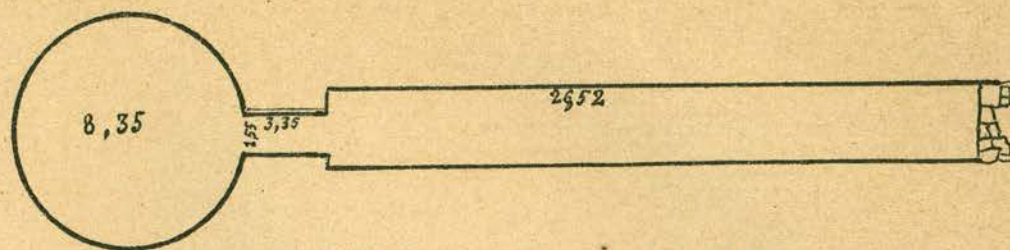
7. Κάτοψι τάφου ἐν Μενιδίῳ.
