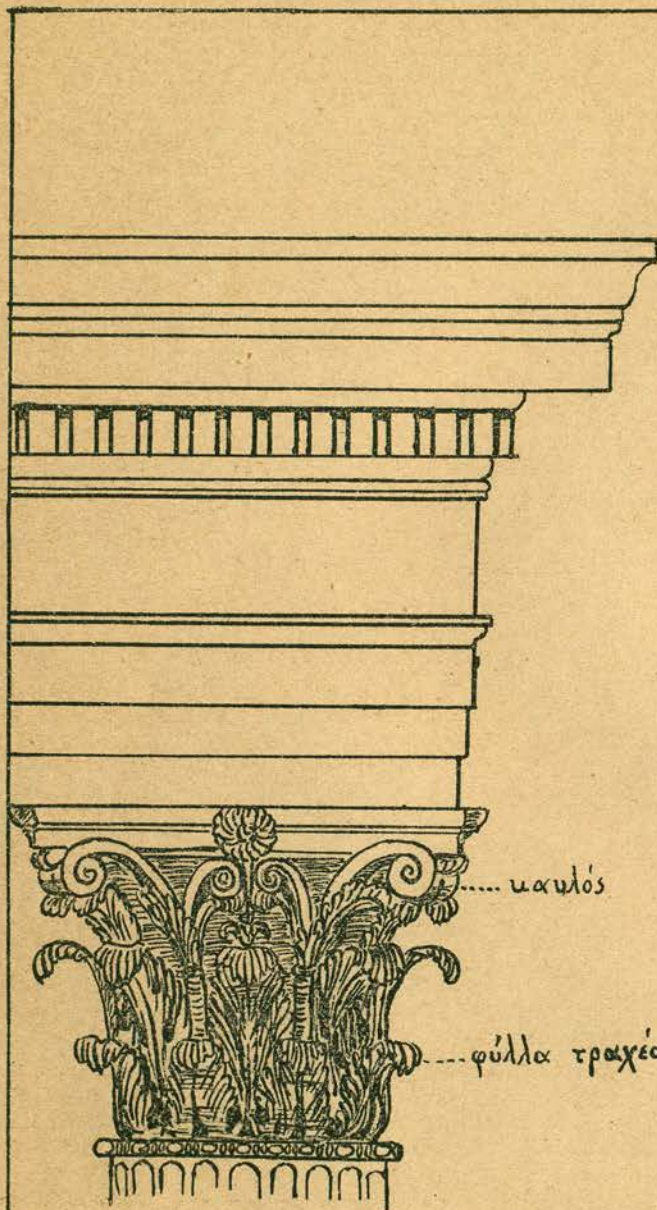
28. Ρυθμός Κόρινθιακός. (ιδ. Vitruv. IV 1,8.)
