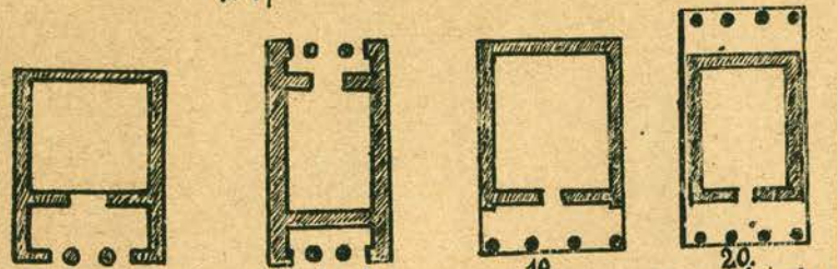
17. Ἐν παραστάσι. 18. Διπλοῦς ἐν παραστάσι. 19. Πρόστυλος. 20. Ἀμφιπρόστυλος
